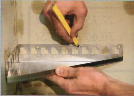
Bohrmarkierungen anzeichnen
